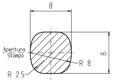
SEZ. MANICO SCALA 3-1
