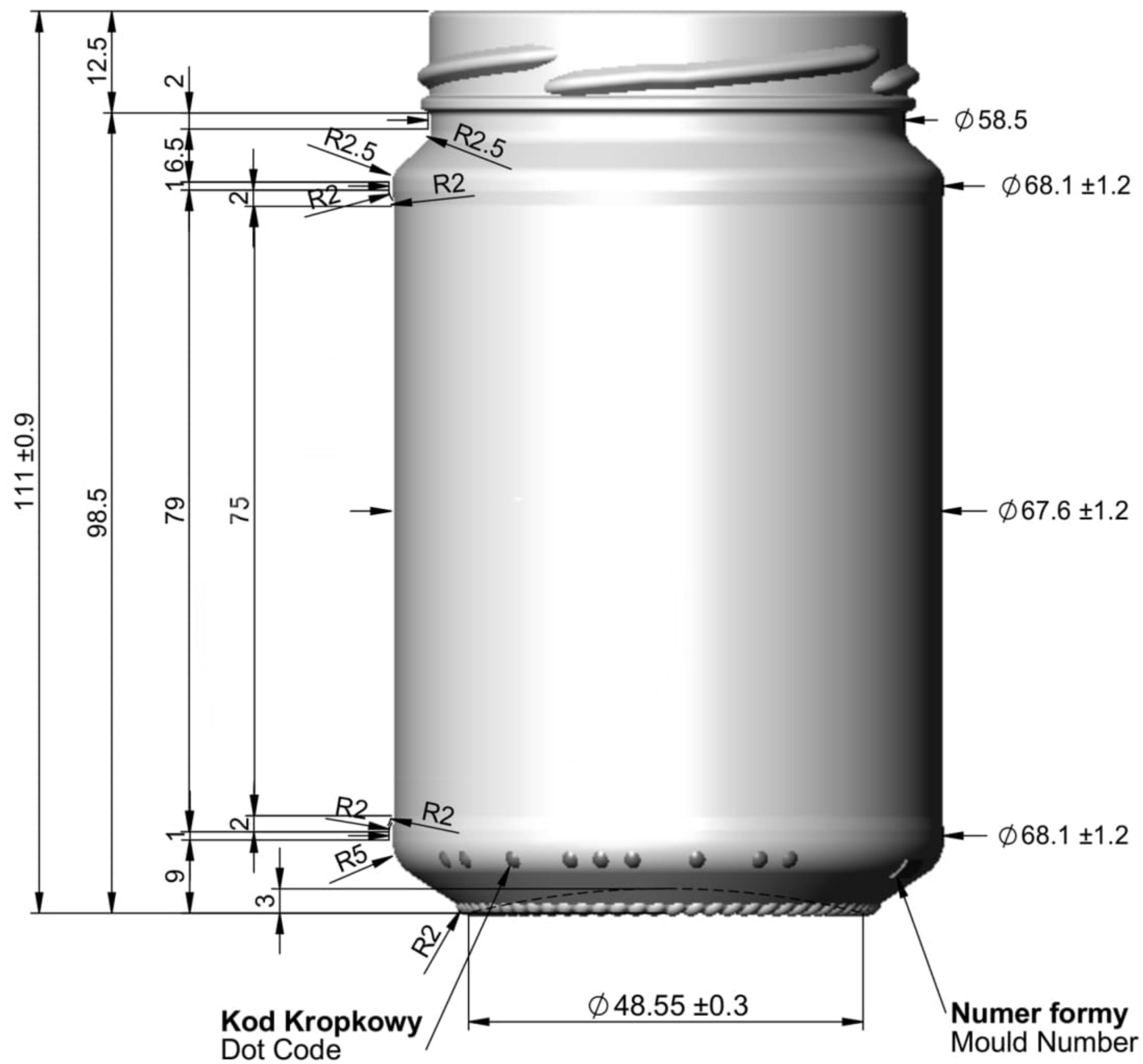
WIDOK Z PRZODU FRONT VIEW
